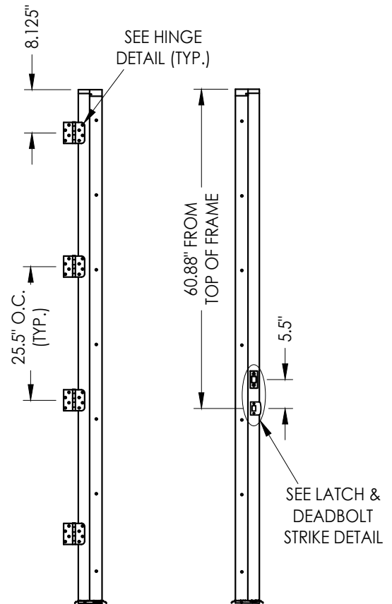
HINGE JAMB
